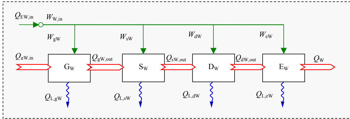
Figura 6 – Schema di calcolo dell'energia primaria per la produzione di acqua calda sanitaria (Fonte: prEN 15316)
